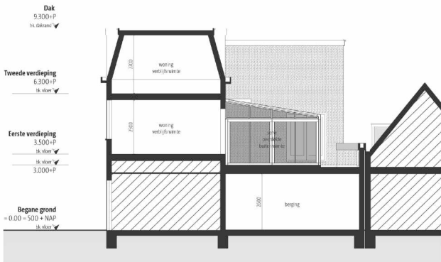
Doorsnede B-B Bestaande situatie
