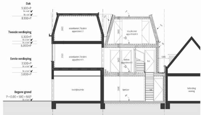
Doorsnede B-B Nieuwe situatie
