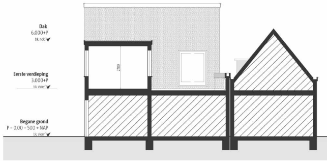
Doorsnede A-A Bestaande situatie
