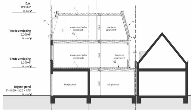
Doorsnede A-A Nieuwe situatie
