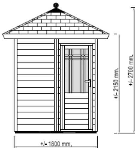
Voor aanzicht Vorder Ansicht Front view
