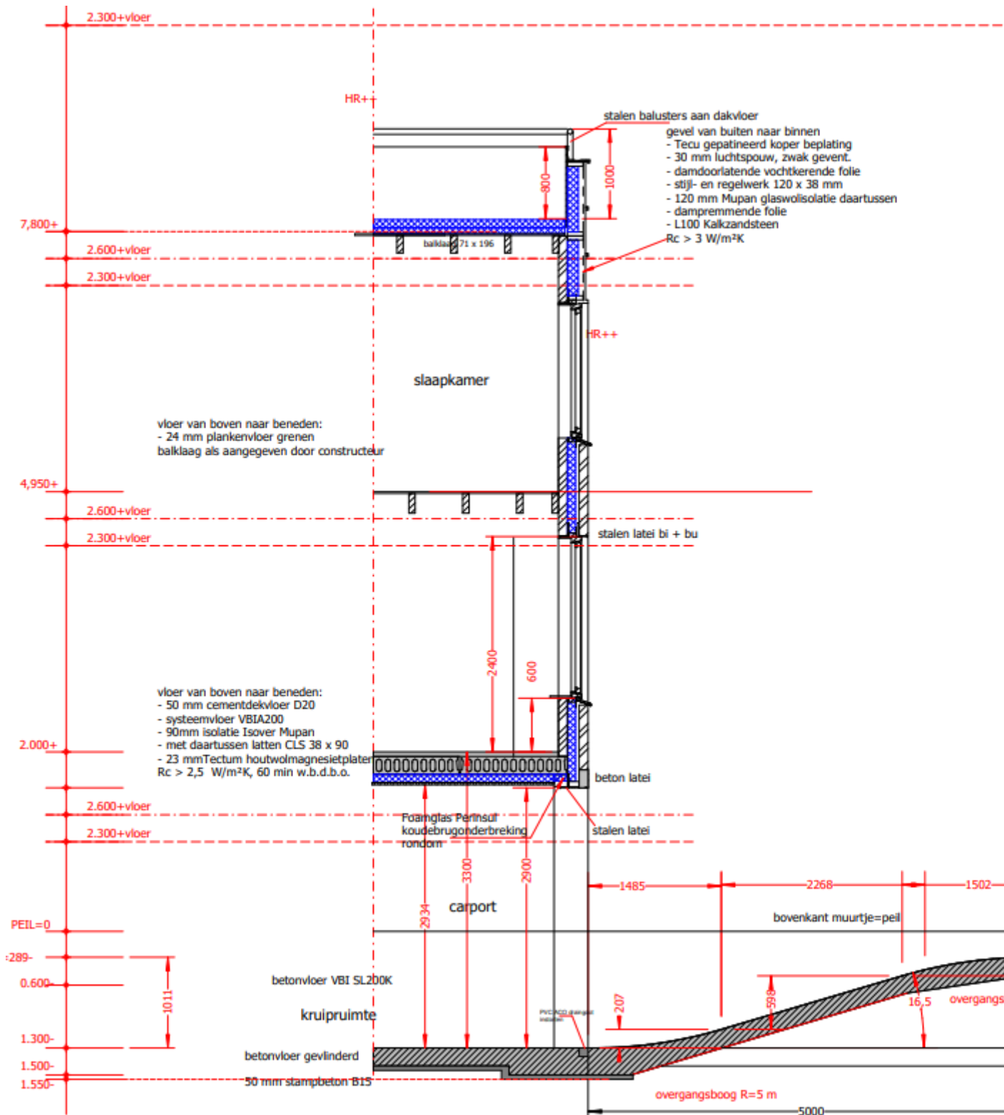
langsdoorsnede B, plan
