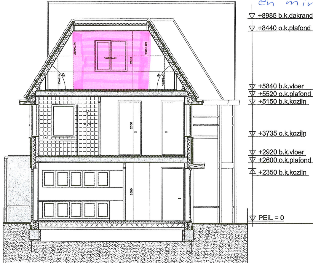
DOORSNEDE C-C
