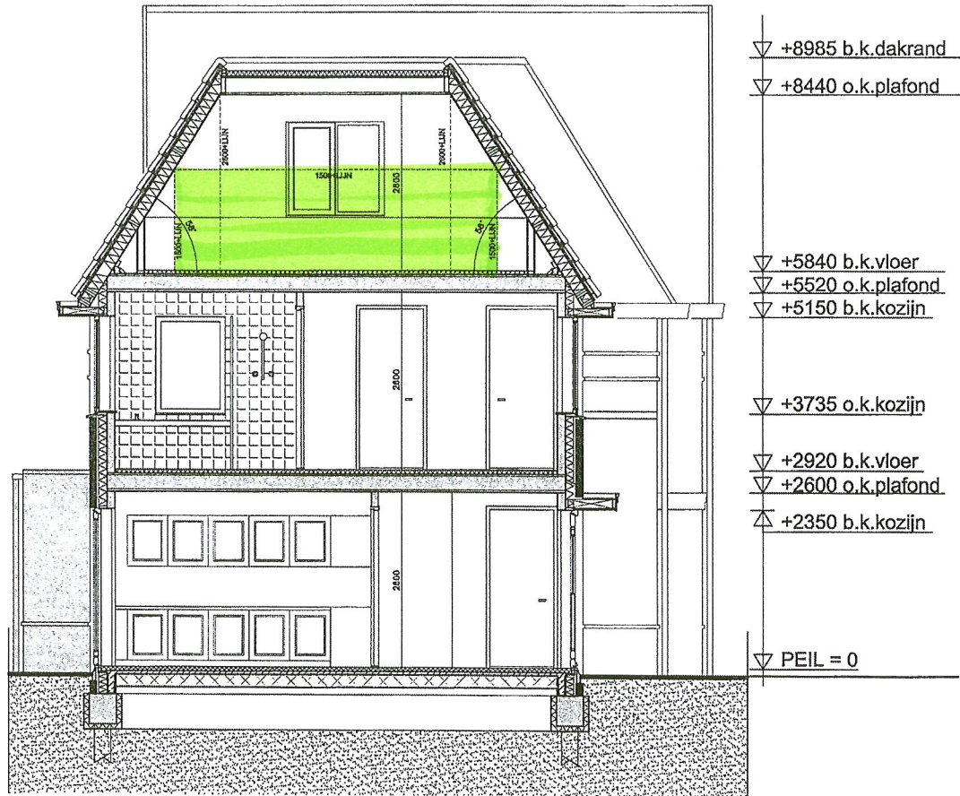
DOORSNEDE C-C
