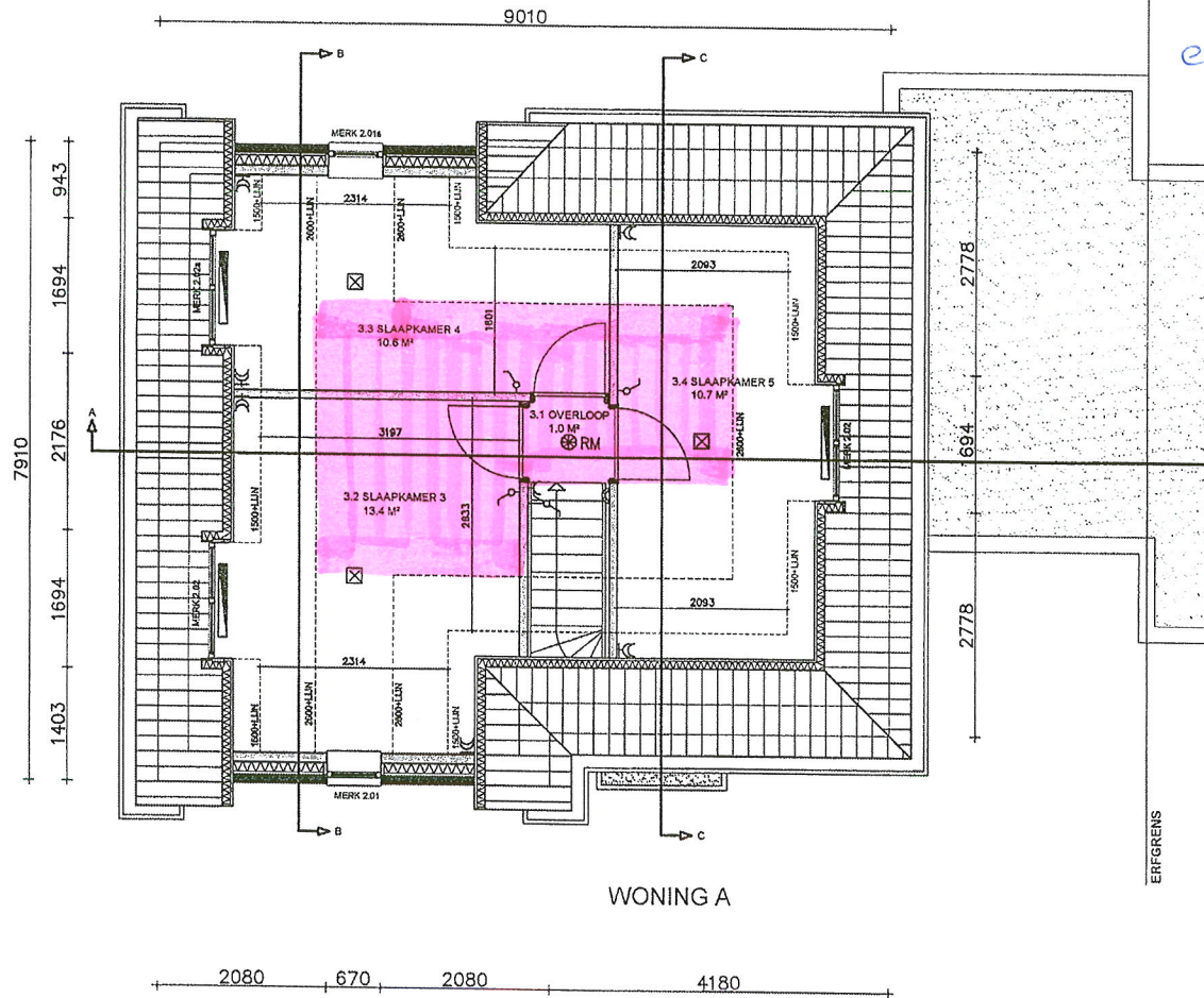
TWEDE VERDIEPING
